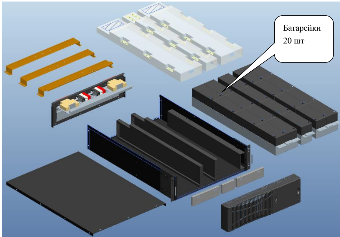
Рис. 4 (Установка 20 шт.)
