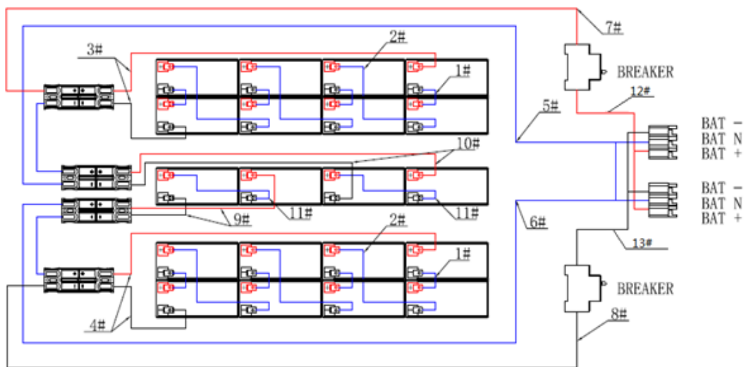
Рис. 4 (Установка 20 шт.)
